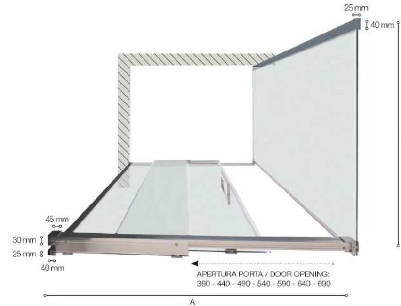
Versione Angolare SX da 1000 mm Left Corner Version 1000 mm
