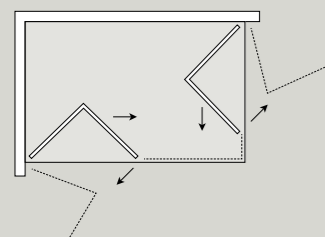
Porta a soffietto Versione: Angolare doppia anta
