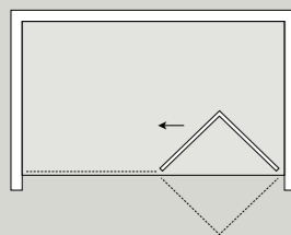
Porta a soffietto Versione: Nicchia
