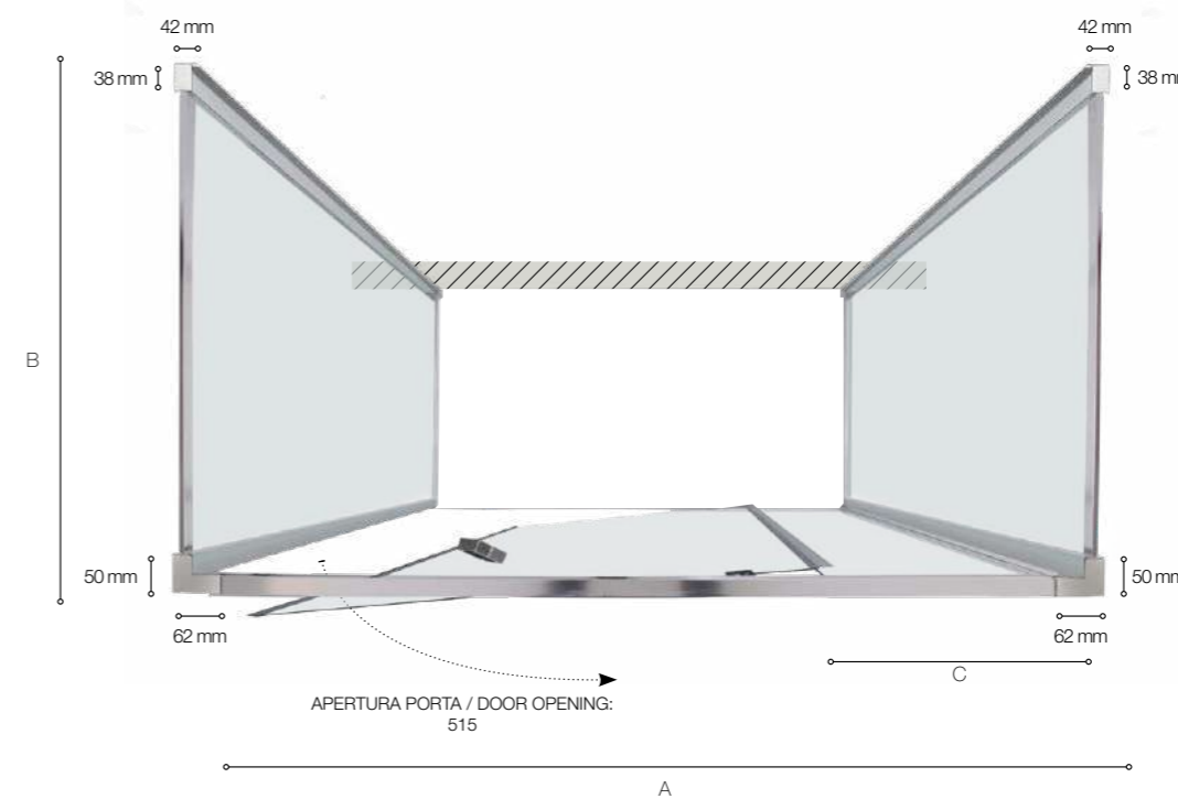
Versione Centro Parete Center Wall Version
