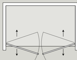
Porta a saloon Versione: Nicchia
