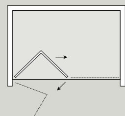
Porta a soffietto Versione: Nicchia
