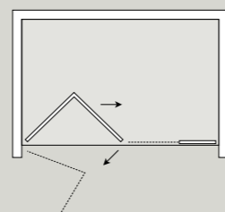
Porta a soffietto Versione: Nicchia
