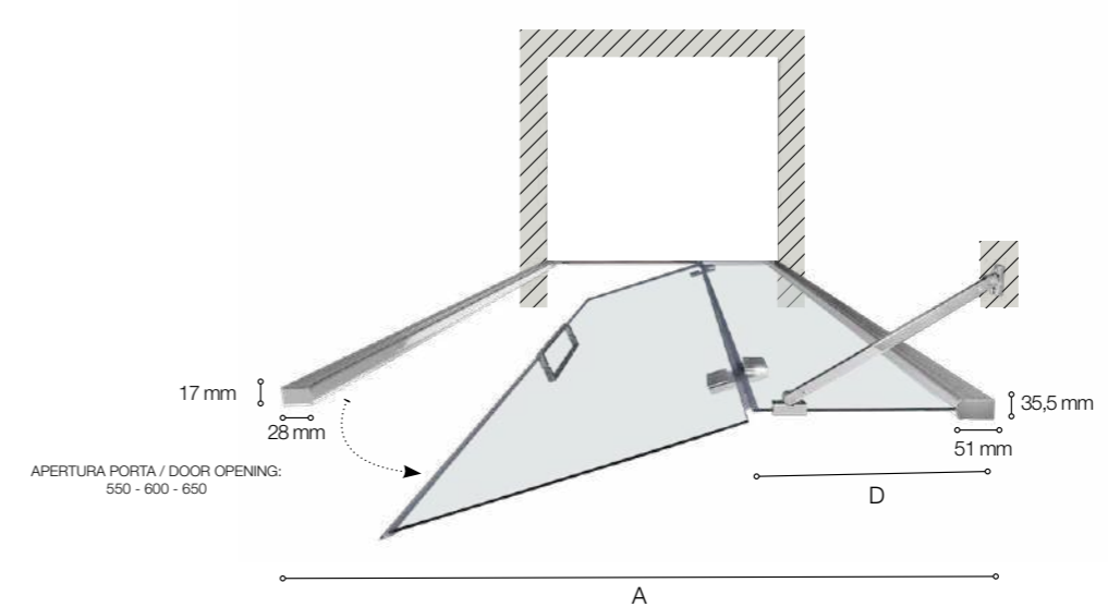
DIMENSIONI PORTA (A) (NICCHIA) CON PROFILO DI CHIUSURA NTPC03 DOOR SIZE (A) (NICHE) WITH CLOSING PROFILE NTPC03
